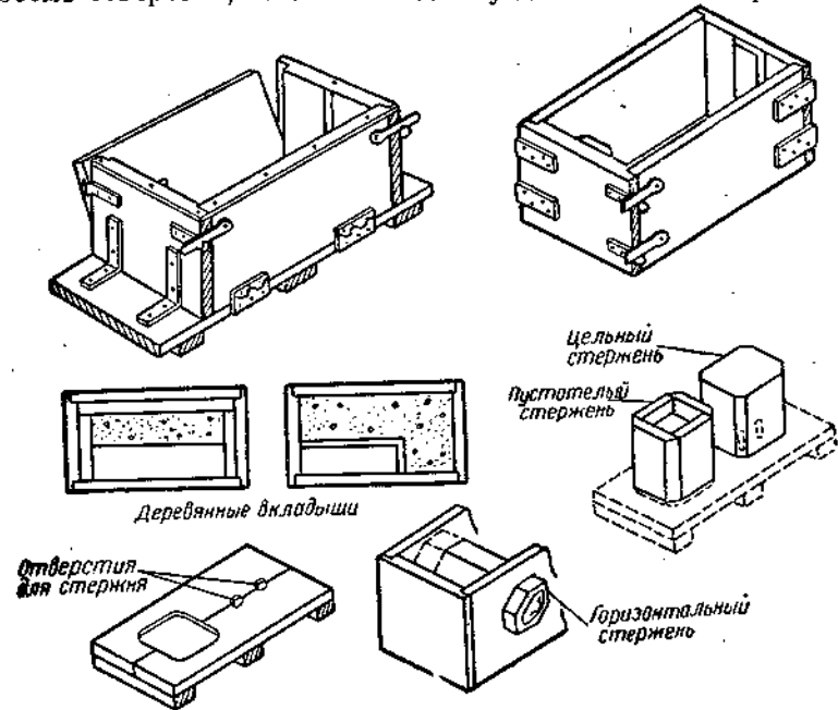
Рис. 123. Деревянные формы и их детали.
