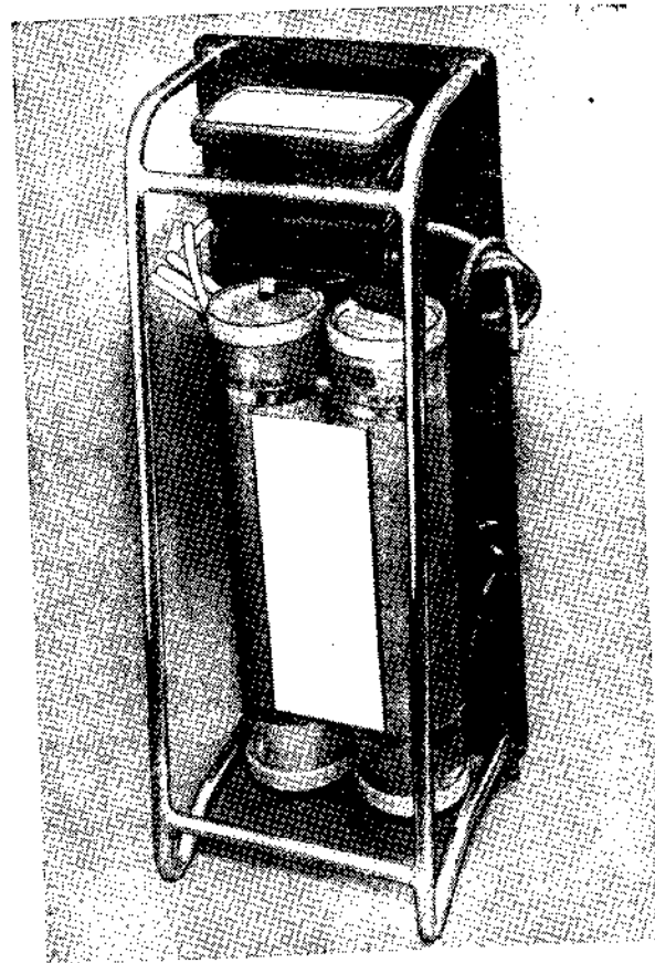
Рис. 1. Установка для деминерализации воды, используемой в лаборатории (фирма «Пермутит», Лондон).
