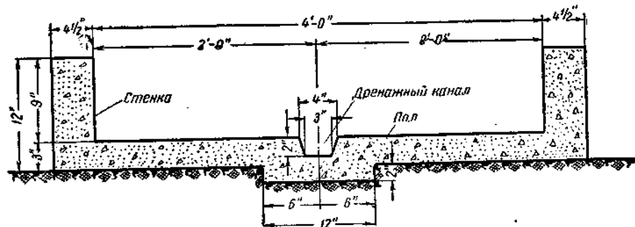
Рис. 83. Поперечный разрез стандартного поддона (длина 15 м).
