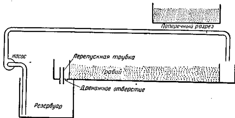
Рис. 2. Голландская гравийная культура.
