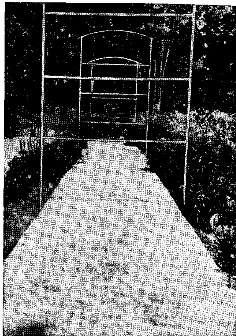
Рис. 93. Деформационные швы в бетонном дне сделаны через каждые 3,75 м. Стены будут сооружены из грунто-цементных блоков.
