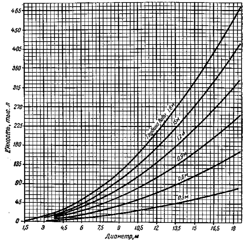
Рис. 118. Диаграмма для определения емкости круглых резервуаров.
