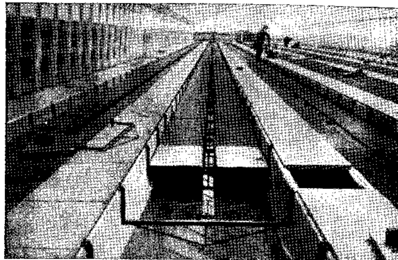
Рис. 95. Наиболее прогрессивный метод строительства поддонов применен в хозяйстве «Электрофлора» (Швеция). Поддоны делают из готовых бетонных плит, металлических распорок и водонепроницаемой полиэтиленовой пленки.
