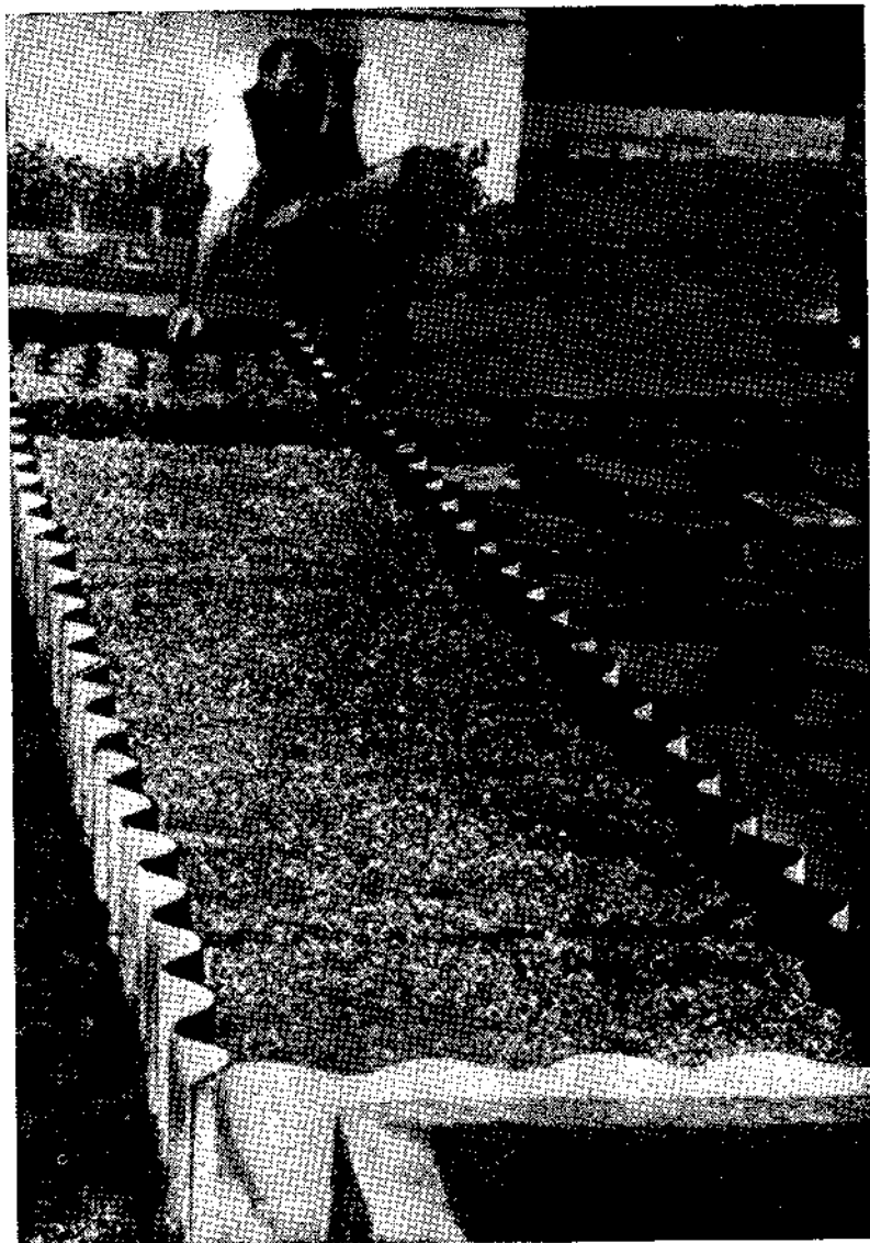
Рис. 107. Поддон из обрезков кровельного эверита толщиной 6 мм. Удобрения применяют в сухом виде.
