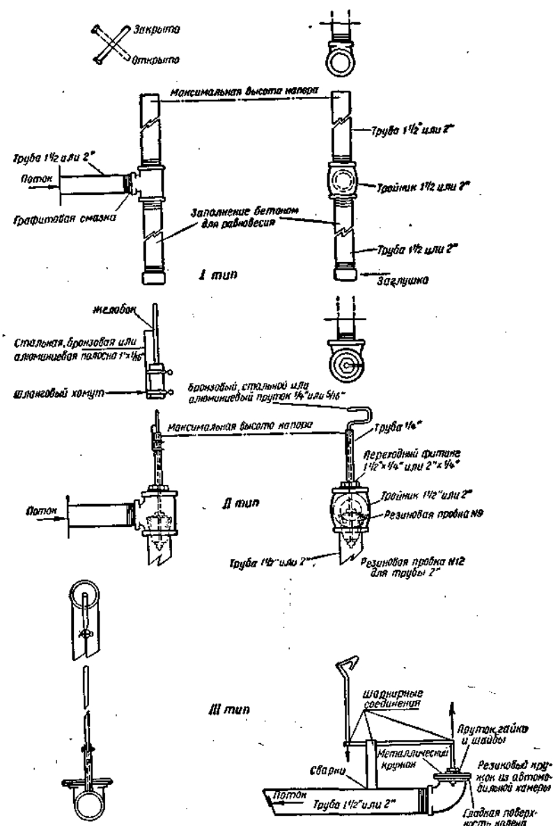
Рис. 104. Три типа клапанов, применяемых в поддонах.
