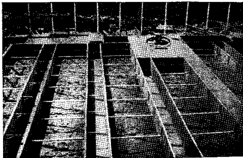
Рис. 96. Основанием служит мягкий песок, на который кладут пленку. Находясь на мягком ложе, пленка не режется и не рвется (хозяйство «Электрофлора»).
