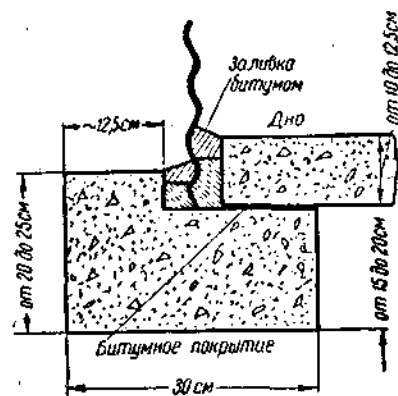
Рис. 124. Соединение стены с дном в резервуарах из разных материалов.
