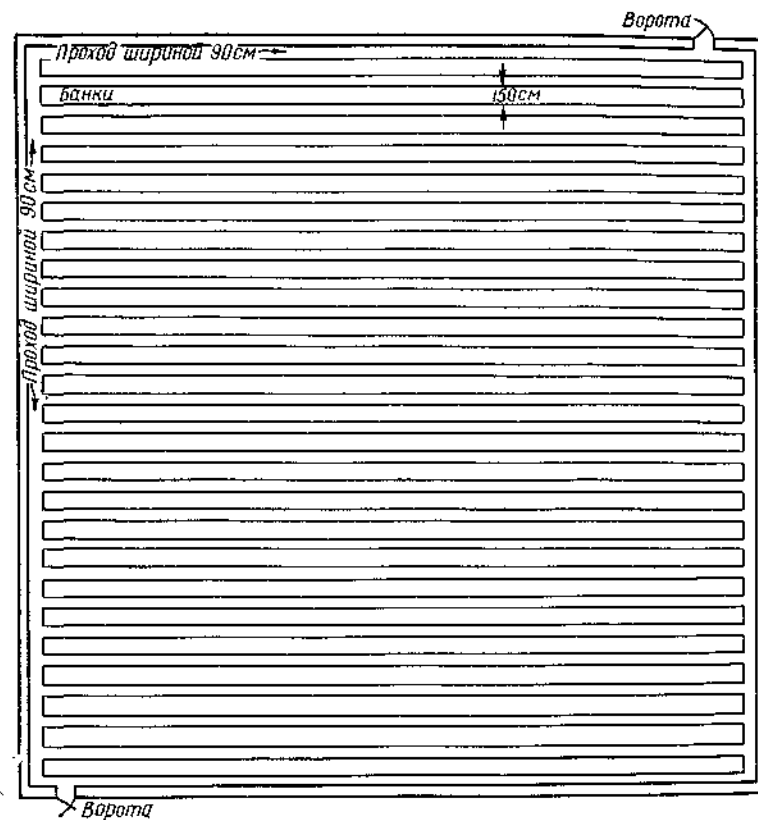
Рис. 108. Общая схема размещения 15 тыс. жестяных банок емкостью 18 л каждая на площади 0,4 га.
