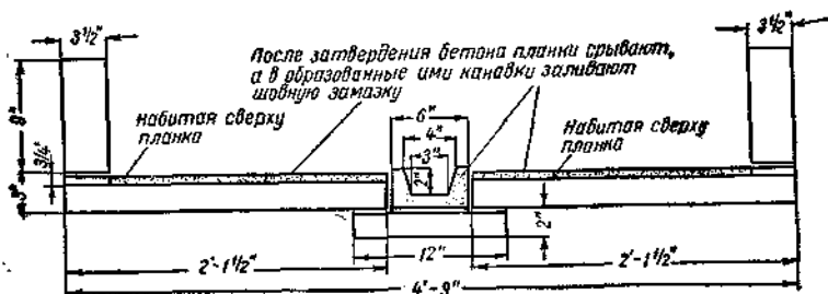
Рис. 87. Чертежи, иллюстрирующие устройство деформационных швов в поддоне.
