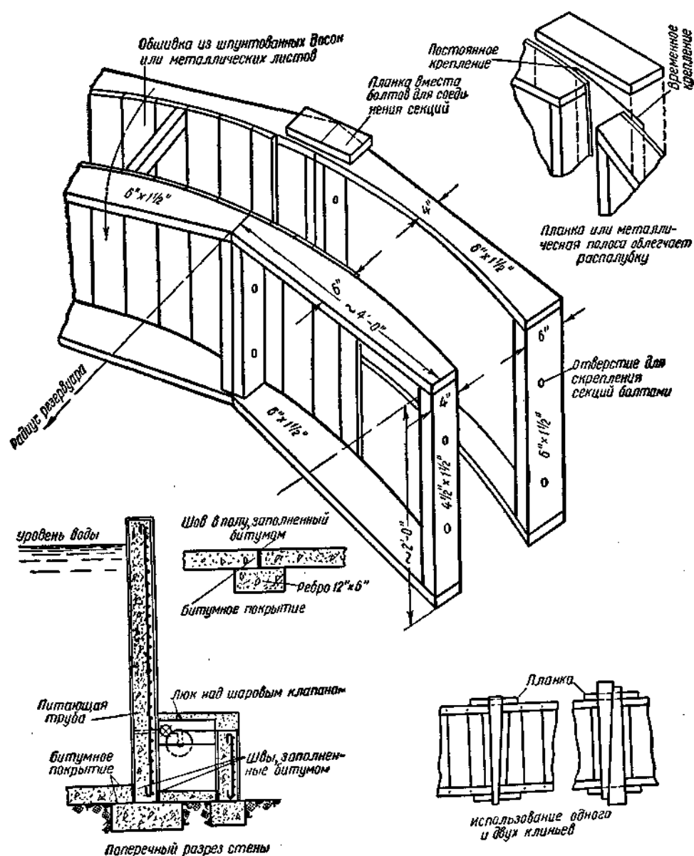
Рис. 120. Опалубка для сооружения круглого бетонного резервуара.
