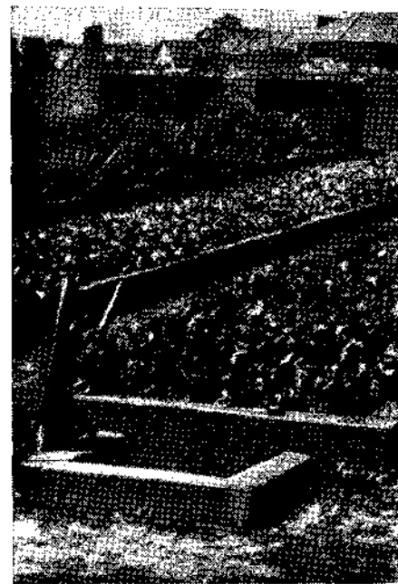
Рис. 81. Крыльчатый насос позволяет экономить время, так как не нужно вручную переносить раствор из приемника в питающий резервуар.
