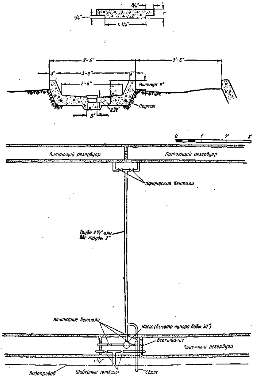
Рис. 103. Трубопроводы и дренаж поддонов.
