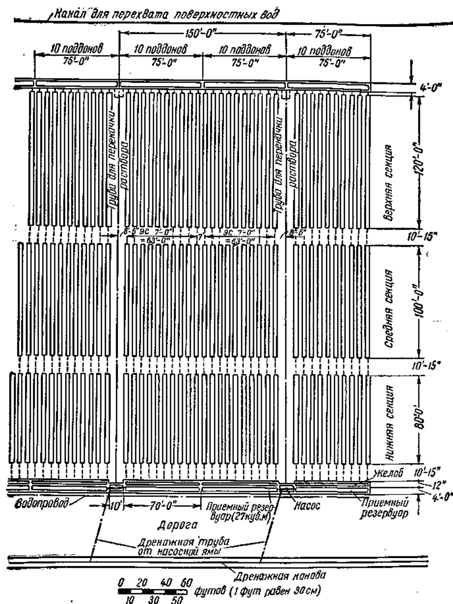
Рис. 101. Схема размещения поддонов при наличии водопроводной сети.
