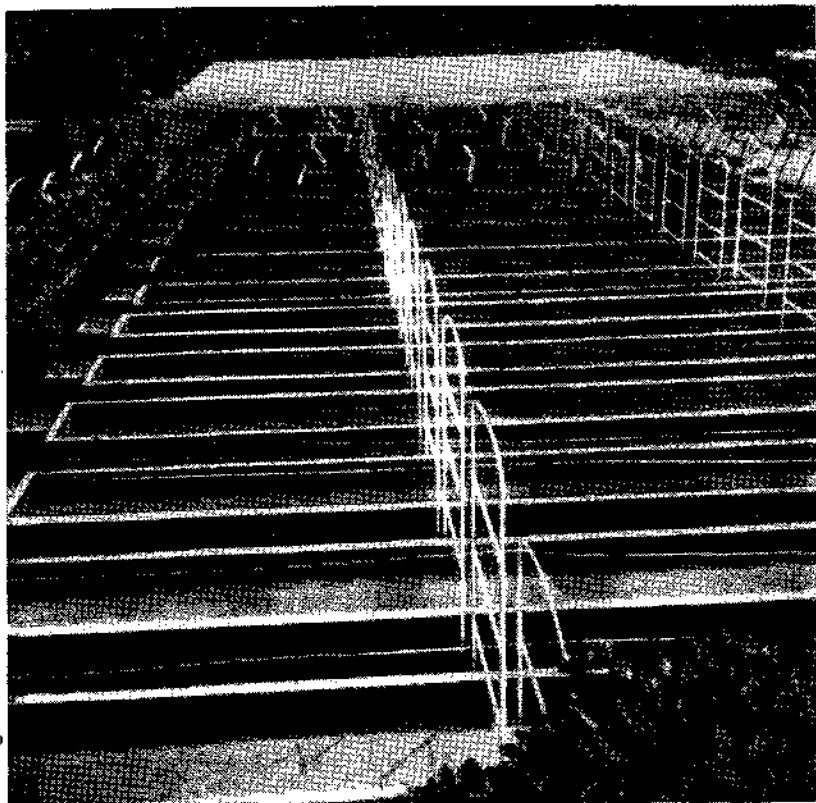
Рис. 67. Поддоны в процессе сооружения. Часть поддонов покрыта пленкой (Замбия).
