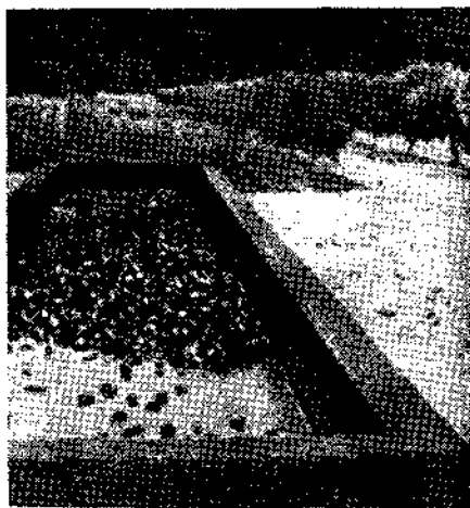
Рис. 73. На дно поддона насыпают 2,5-сантиметровый слой гравия, который разравнивают садовыми граблями. Поддон оштукатурен изнутри и снаружи и покрыт двумя слоями битумной краски фленткот.
