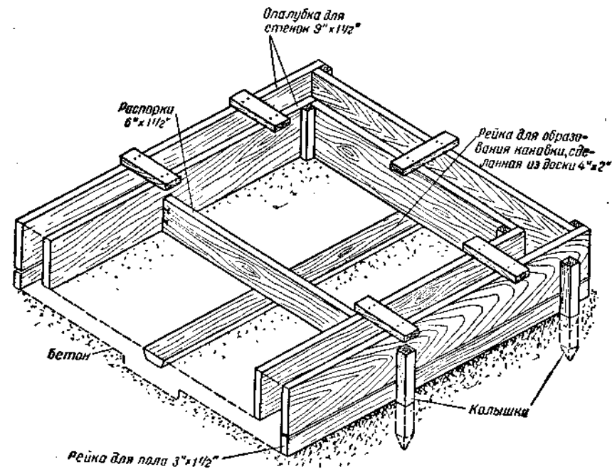
Рис. 84. Общий вид части опалубки для сооружения поддона.
