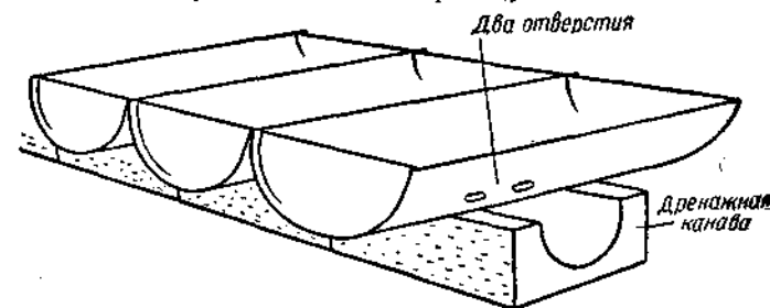
Рис. 112. Схема размещения бочек на бетонном желобе.
