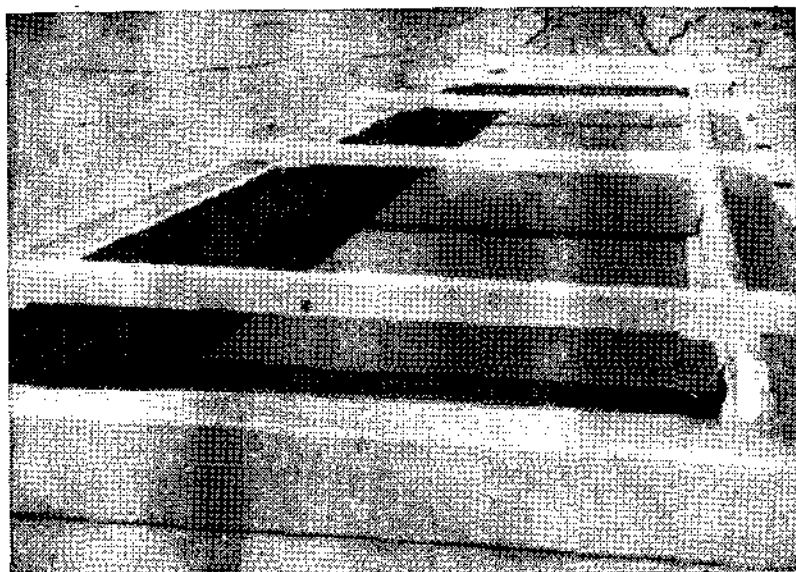
Рис. 92. Опалубка, заполненная бетоном.
