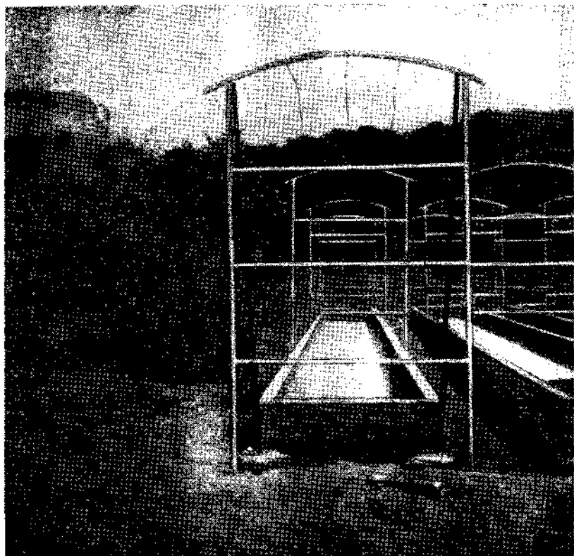
Рис. 82. Готовые для заполнения субстратом поддоны. В левом верхнем углу виден круглый кирпичный резервуар для питательного раствора (Замбия).
