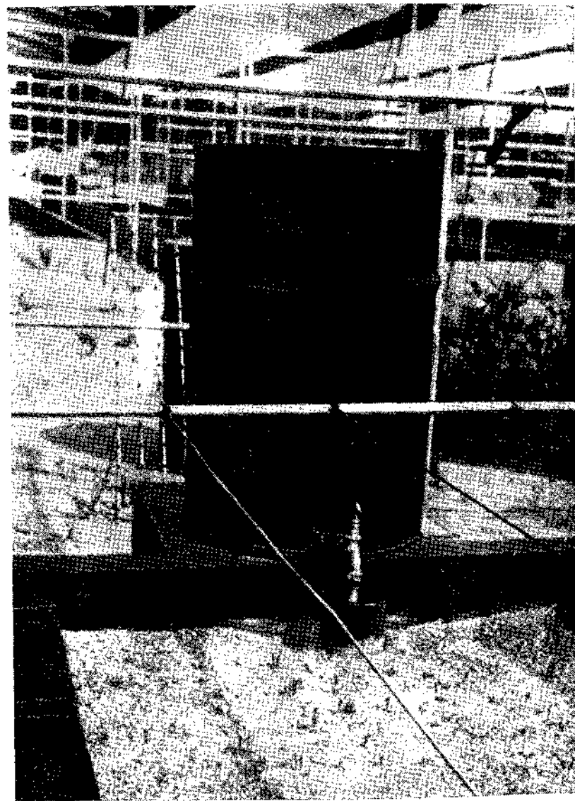
Рис. 70. Если раствор поступает в широкую трубу, опирающуюся одним концом на дно поддона, то можно наблюдать за уровнем раствора в субстрате. Это очень важно в тропических районах, где влага испаряется очень быстро. Резервуары и трубы следует покрыть двумя слоями битумной краски флинткот.
