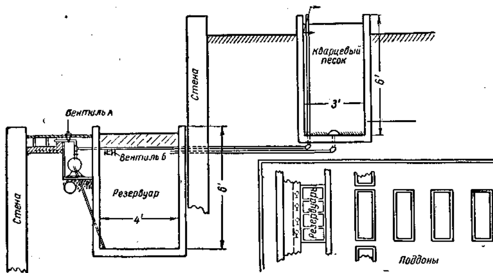
Рис. 113. Схема гидропонника для выращивания деревьев.
