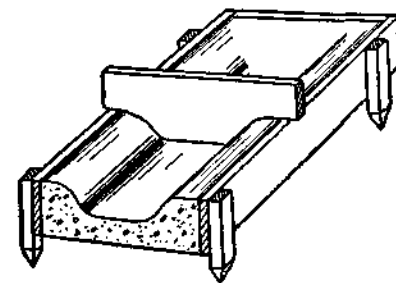
Рис. 119. Бетонная канавка для сброса воды.
