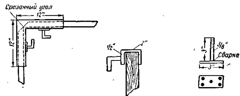
Рис. 91. Крепление углов опалубки.
