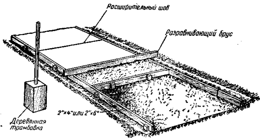
Рис. 117. Укладка бетона на горизонтальную поверхность.
