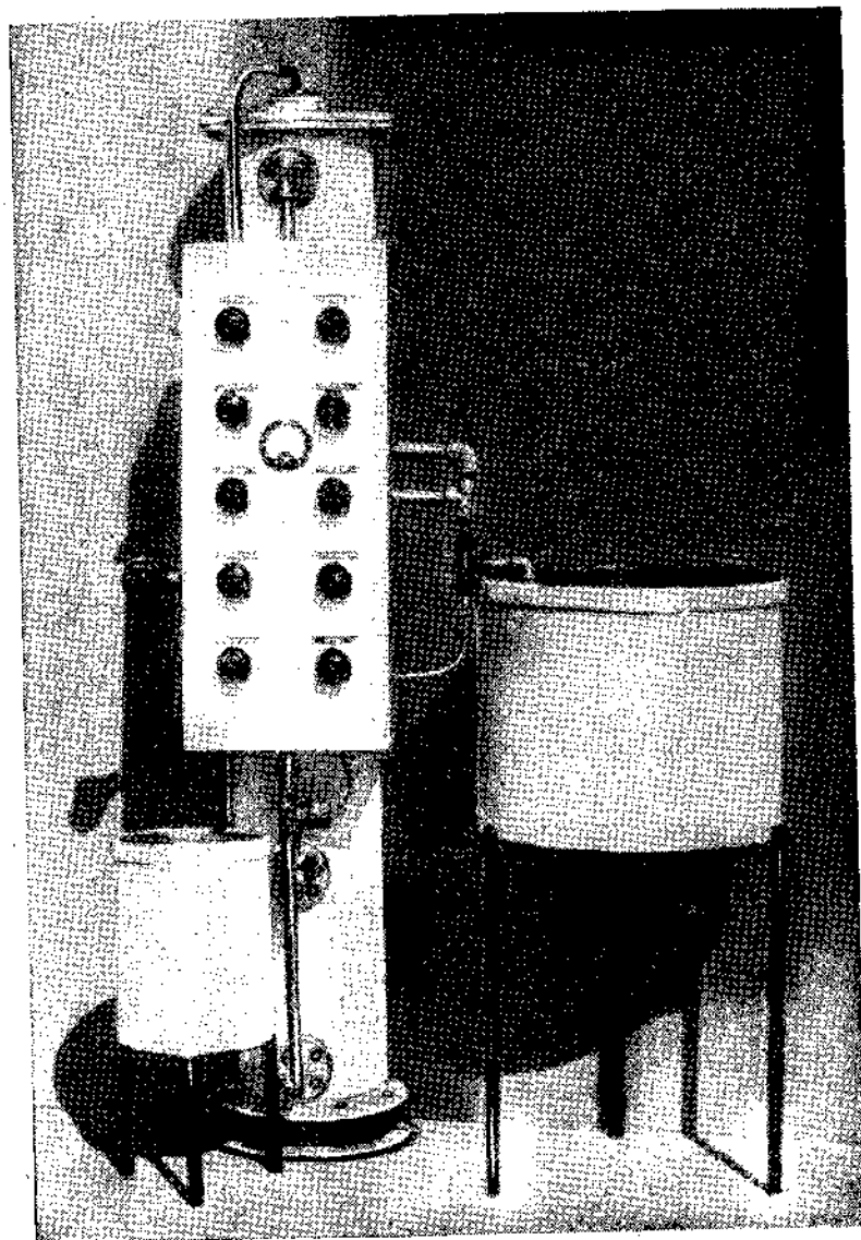
Рис. 125. Современная установка «Пермутит» для очистки шахтных вод.
