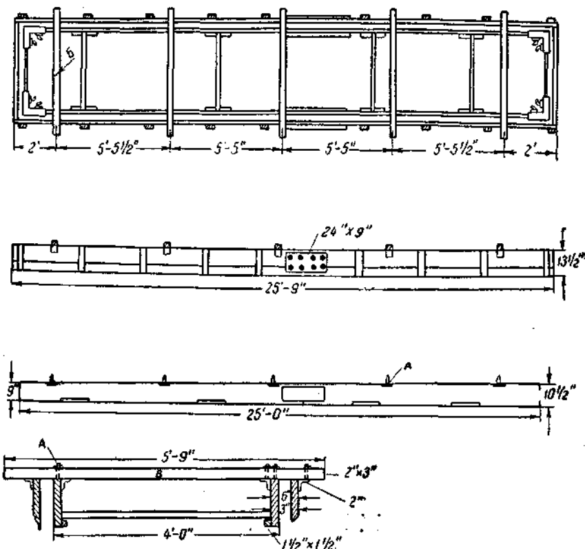
Рис. 90. Опалубка, применяемая в пустыне Калахари.
