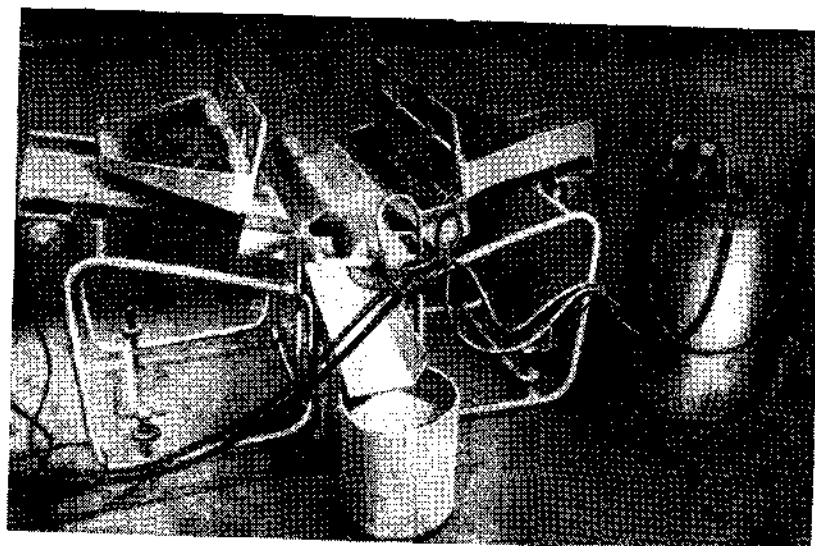
Рис. 116. Переносная печь для обжига вермикулита.
