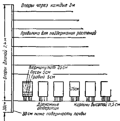
Рис. 110. По экономическим соображениям в банках следует выращивать высокорослые растения. На схеме показано устройство опор для таких культур, как помидоры.
