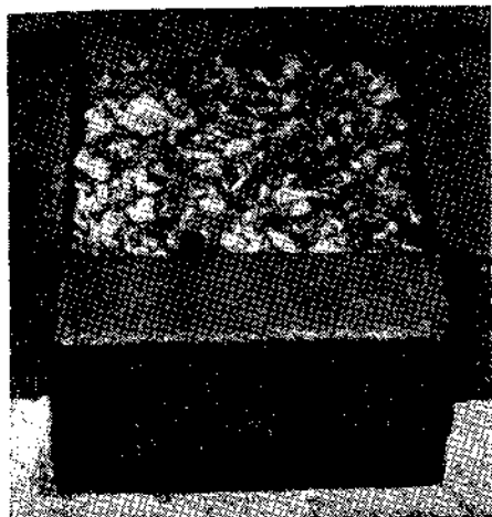
Рис. 71. 15-сантиметровый слой гравия с частицами диаметром 13 мм насыпан для дренажа между кирпичами перед выпускным отверстием внутри поддона.
