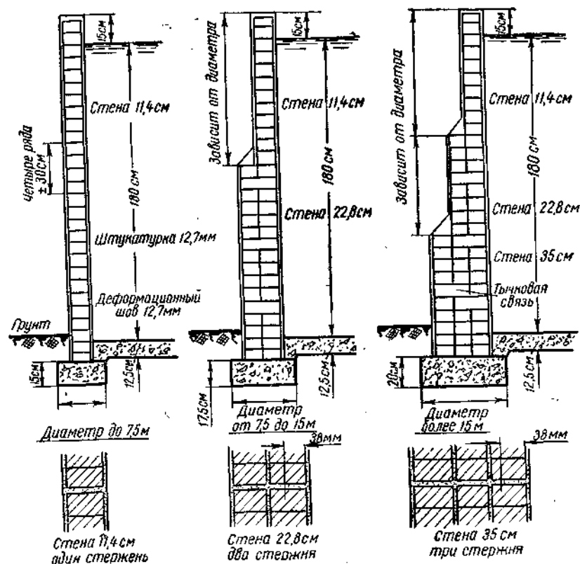
Рис. 121. Разрез кирпичной стены круглого резервуара.
