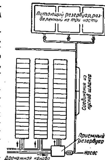
Рис. 111. Схема размещения 200-литровых бочек.
